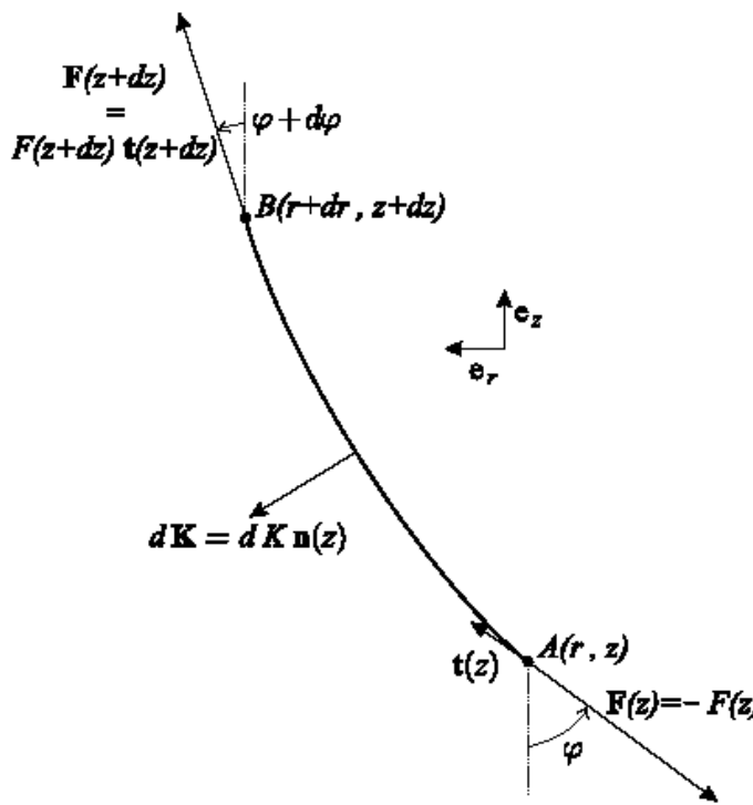
Figure 6 - Représentation des forces s'exerçant sur une longueur élémentaire d\ell = AB du filin
