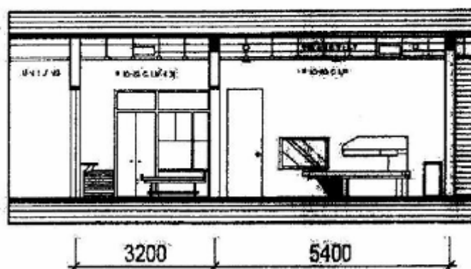
MẶT CẮT
