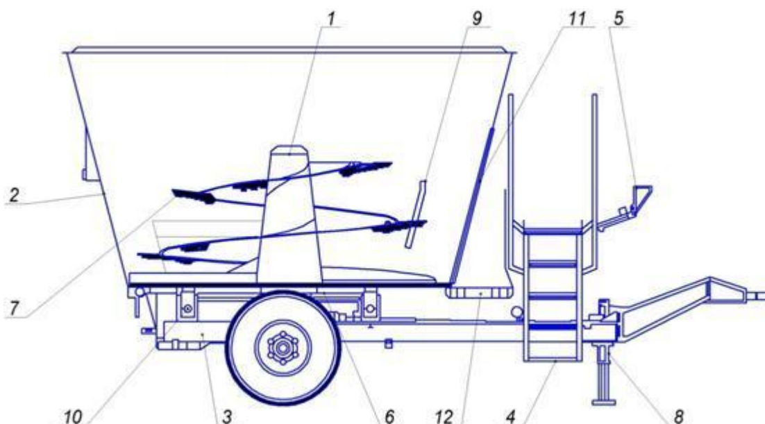
Рис. 5.6. Схема комбінованого агрегату для приготування і роздавання кормів: 1 - робочий орган (ротатор, шнек); 2 - бункер; 3 - рама; 4 - оглядова драбина; 5 - дисплей системи зважування;
