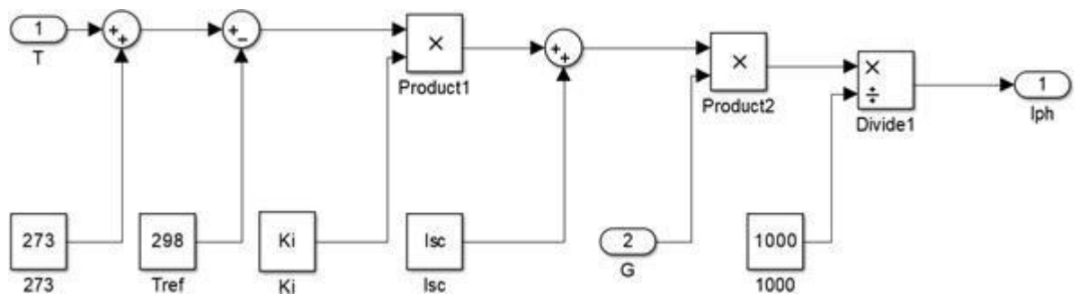
Hình 5.4: Dòng quang điện của pin mặt trời
