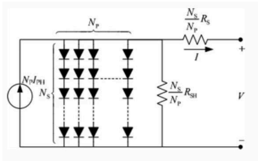
Hình 1.5: Sơ đồ nhiều tế bào quang điện của pin mặt trời. Dòng điện của pin mặt trời có N_p tế bào song song và N_s tế bào nối tiếp
