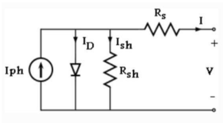
Hình 1.4: Sơ đồ tương đương pin mặt trời.
