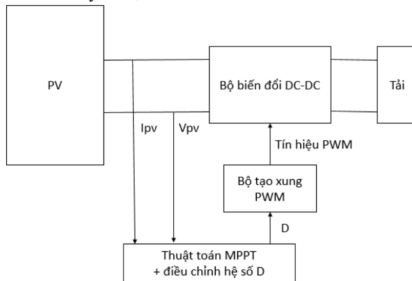
Hình 2.14: Sơ đồ khối phương pháp điều khiển trực tiếp MPPT Tổng trở của PV được coi là tổng trở vào bộ biến đổi. Nhắc lại công thức (2.6):
