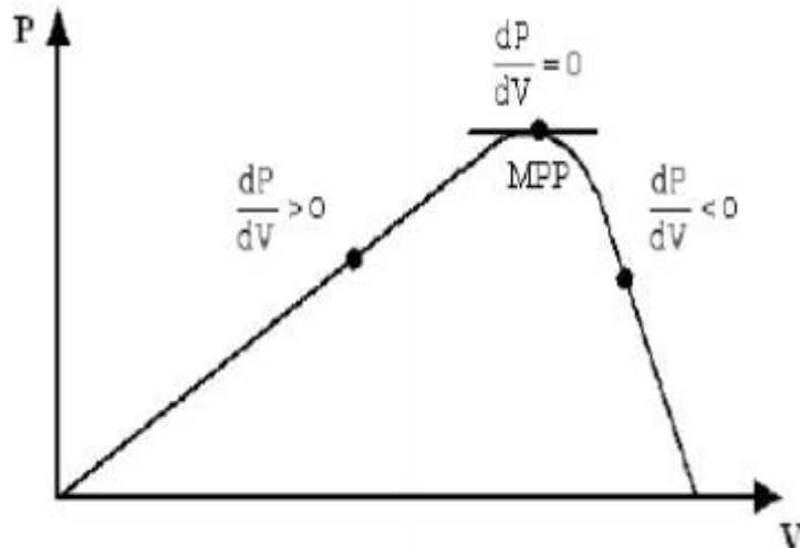
Hình 1.17: Phương pháp điện dẫn gia tăng
