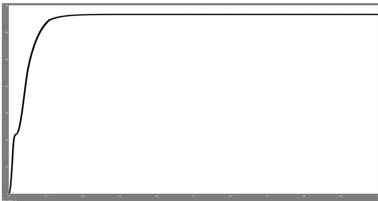
Hình 5.13: Công suất ra của tấm pin với thuật toán P&O (66W)
