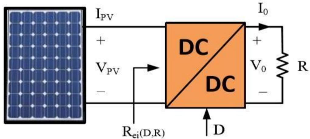
Hình 2.4: Pin mặt trời nối với tải qua bộ biến đổi DC-DC
