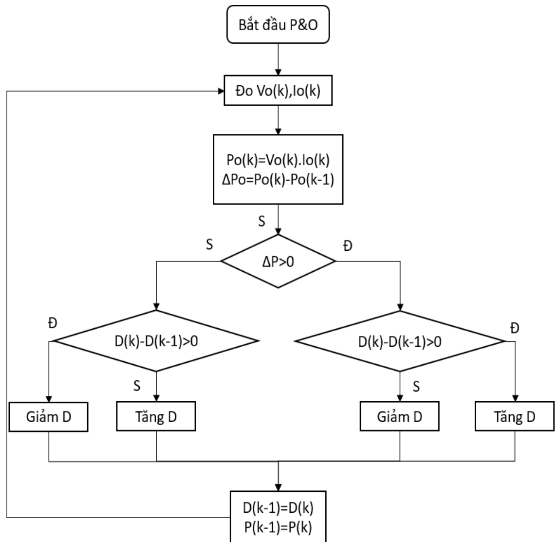
Hình 2.18: Lưu đồ thuật toán P&O điều khiển trực tiếp tín hiệu ra
