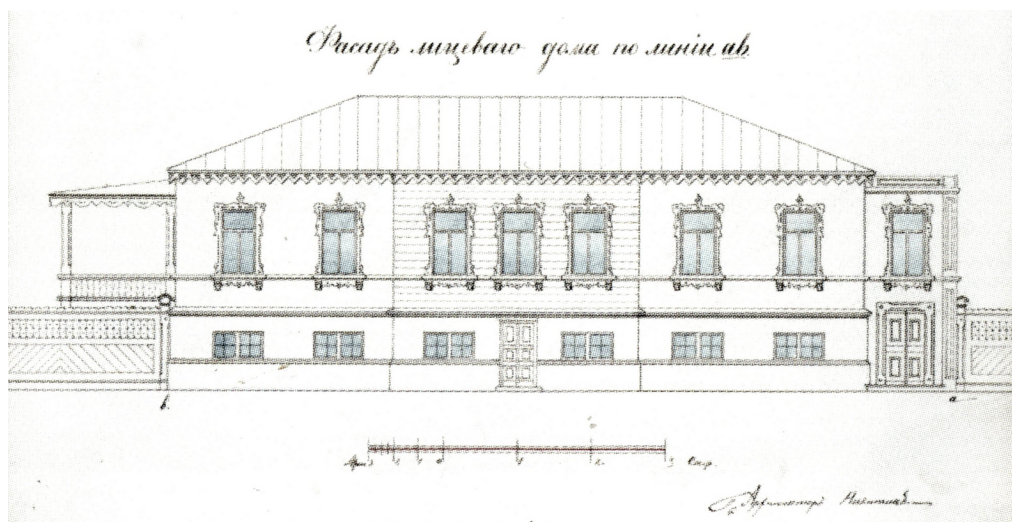
Фасад лицевого дома по линии а б с предполагаемыми изменениями
