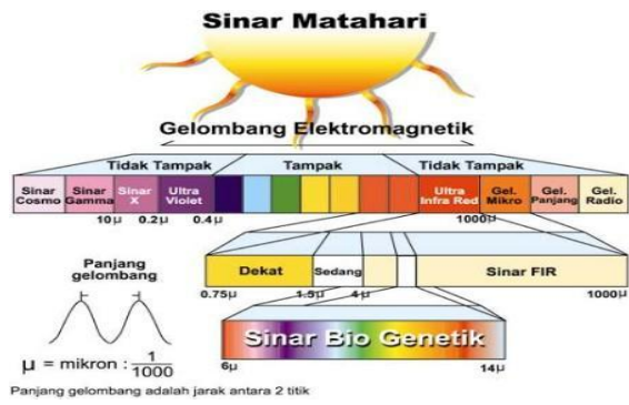
Gambar 1. Sinar yang Dihasilkan Matahari Sumber: Andang Sunarto (2013)
