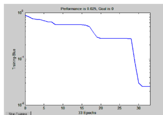
Gambar 1. Grafik Pelatihan Jaringan Syaraf Tiruan
