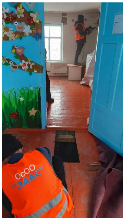
Фото 21. Фрагмент вскрытия пола корпуса №2
