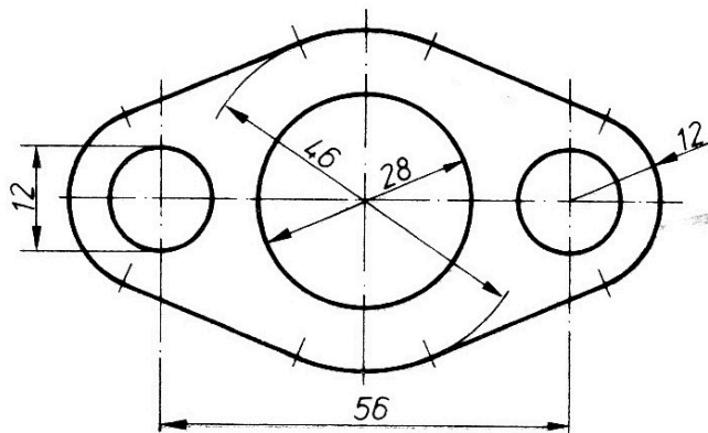
Fig. 19.5 Cubrejunta.
