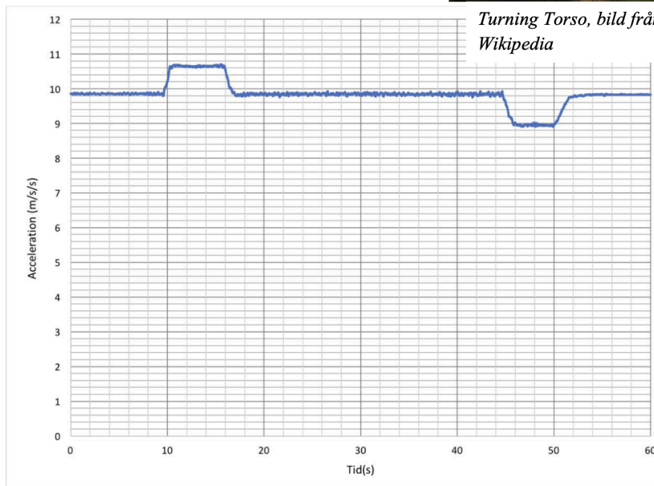
Diagram uppmätt med accelerometern i en mobiltelefon vid en hissfärd i Turning Torso.
