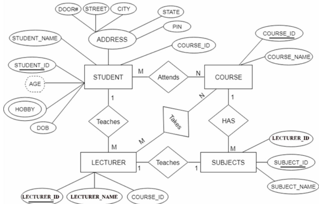
Figure 5.1: ER diagram
