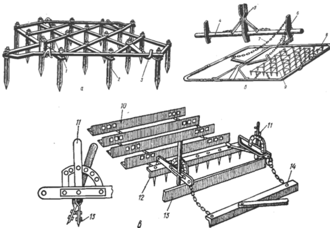
Рис. 2. Борони зубові:
