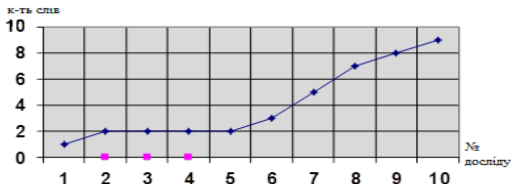
Рис.1.1 Крива пам'яті
