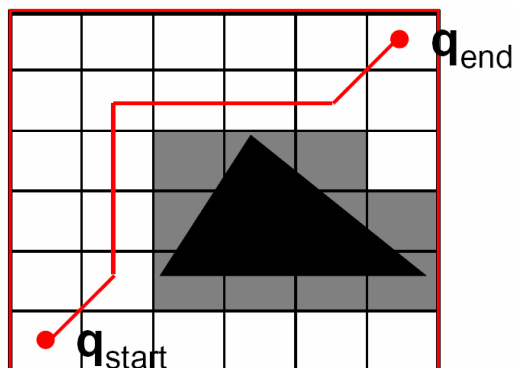
Рис. 8. Решение задачи с помощью разбиения пространства на регулярные клетки
