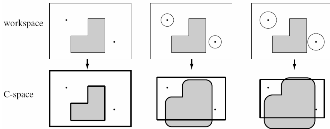
Рис. 4. Получение C_{obs} в явном виде
