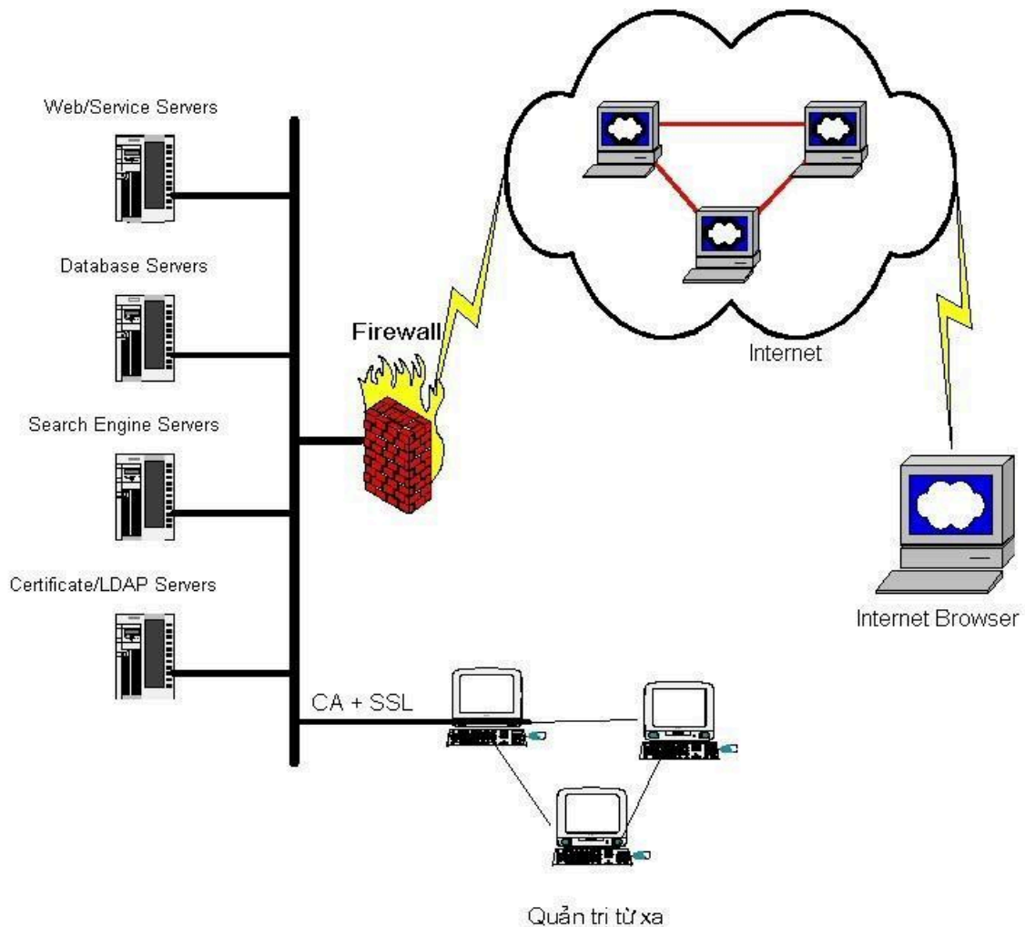
Hình 21.1: Mô hình Web nói chung
