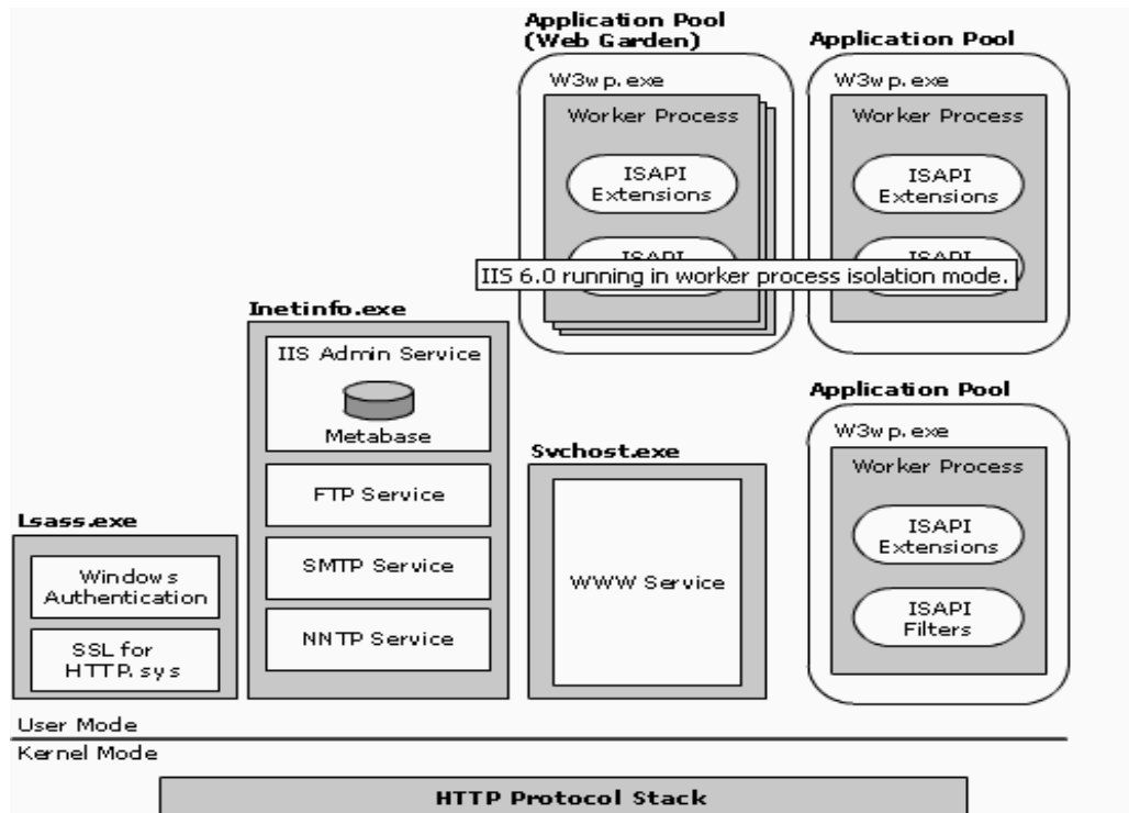
Hình 21.3: Kiến trúc của IIS 6.0 chạy trên chế độ Worker Process Isolation.
