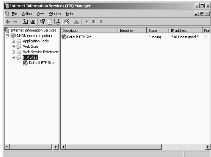
Hình 21.45 IIS Manager.
