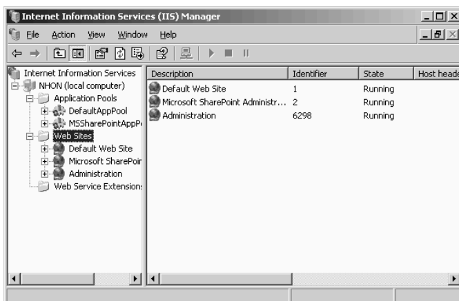
Hình 21.14 IIS Manager.
