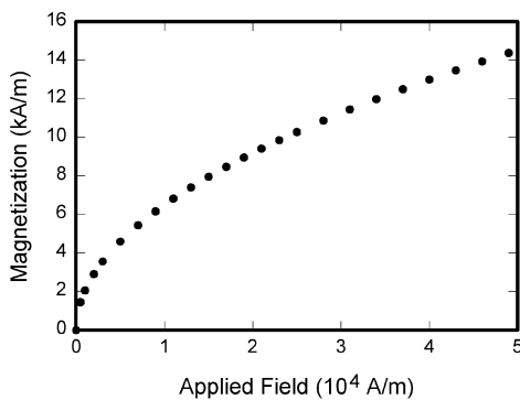
Gambar. 1. Magnetisasi sebagai fungsi yang teraplikasikan. Berikan judul gambar yang jelas dan deskriptif (9).
