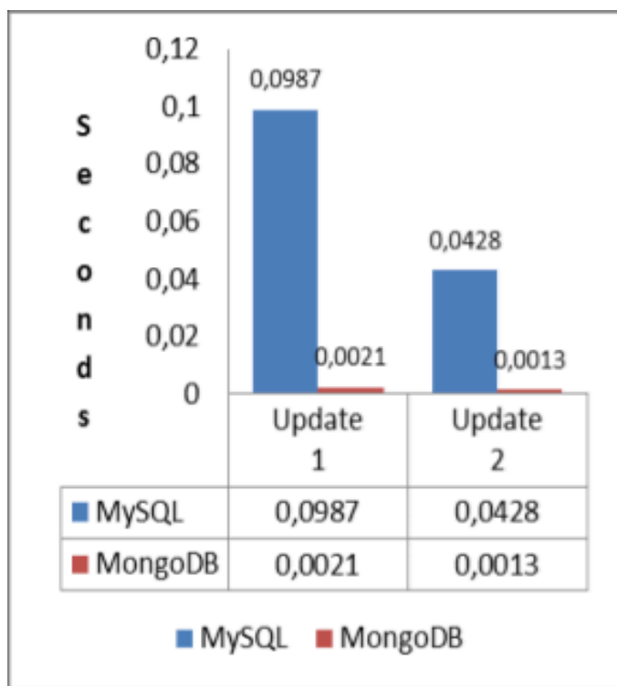
زمان بروز رسانی اطلاعات - my sql & mogodb
