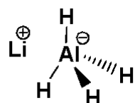
L'hydrure de lithium et d'aluminium
