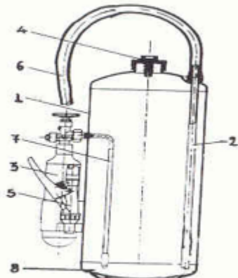
Πυροσβεστήρας ξηράς σκόνης με εξωτερικό φιαλίδιο CO 2
