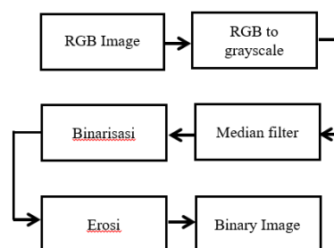
Gambar 1. Tahapan praproses
