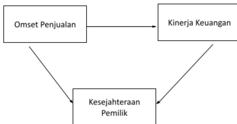
Gambar 4. Kerangka Konseptual
