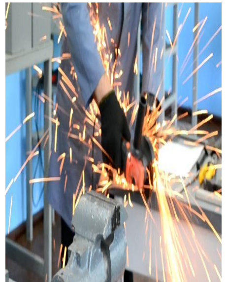
6. Зрізаємо залишки металу і вирізаємо заготовку по кресленню
