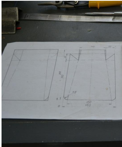
1. Креслення металевого совка
