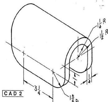
FIG. 5-65 Edge protector.
