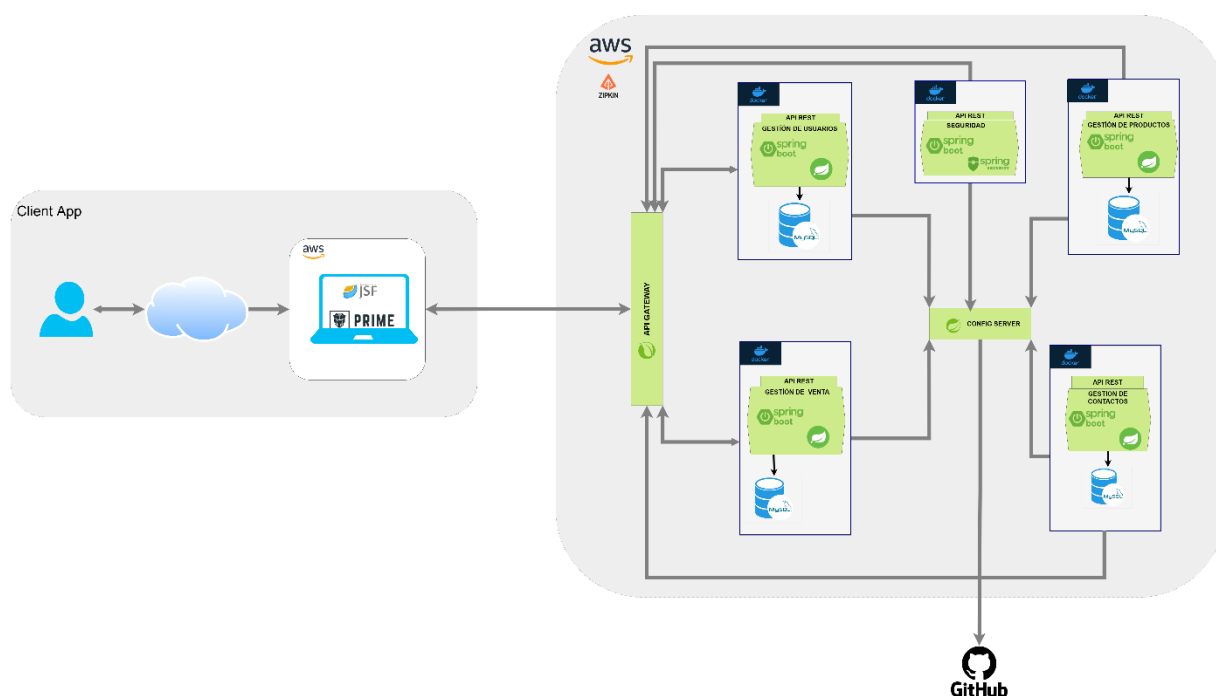
Ilustración 4 Arquitectura de Implementación.
