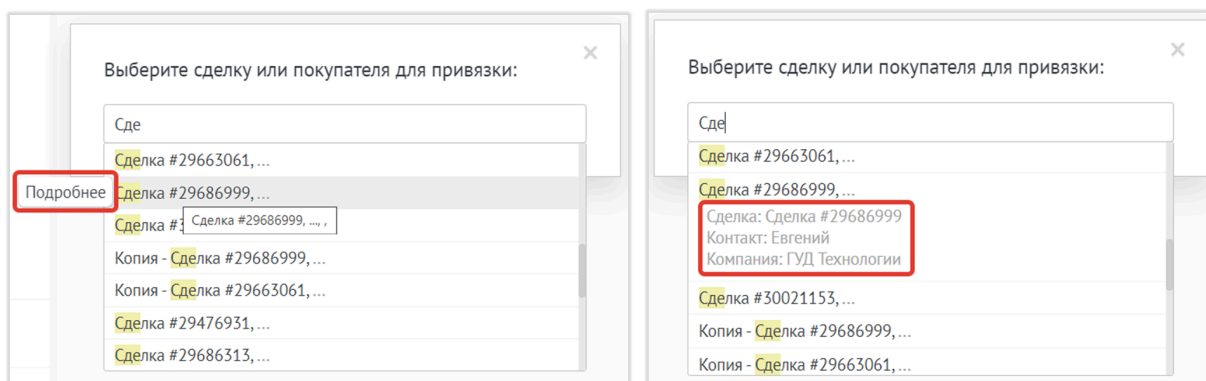
Рис. 7. - Список сделок с подробной информацией
