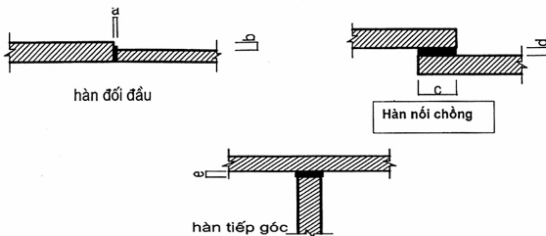
Hình 1 - Các kiểu hàn
