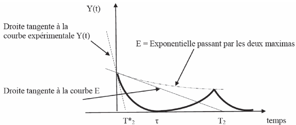
Figure 9 - Enveloppe du signal reçu
