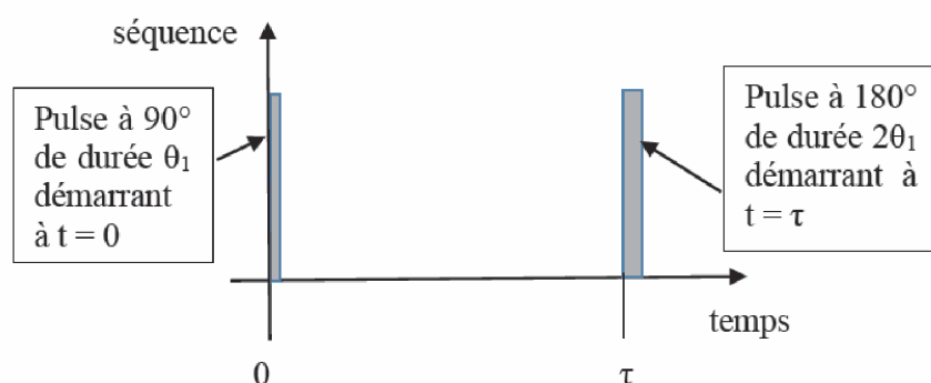
Figure 7 - Écho de spin
