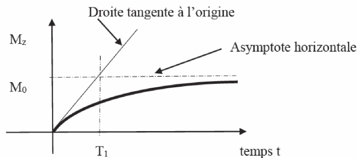
Figure 2 - Relaxation longitudinale
