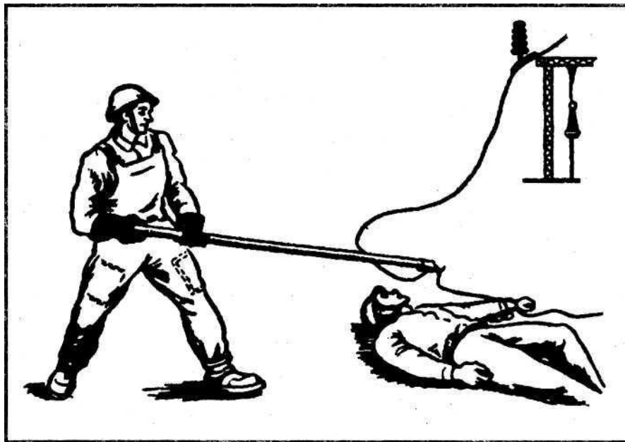
Рис. 23. Звільнення потерпілого від дії струму в установках понад 1000 В відкиданням проводу ізолюваною штангою
