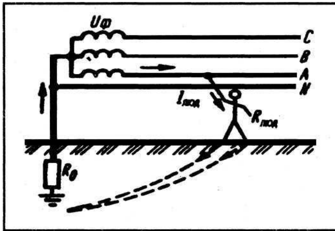
Рис. 16. Однофазне дотикання в мережі з глухозаземленою нейтраллю
