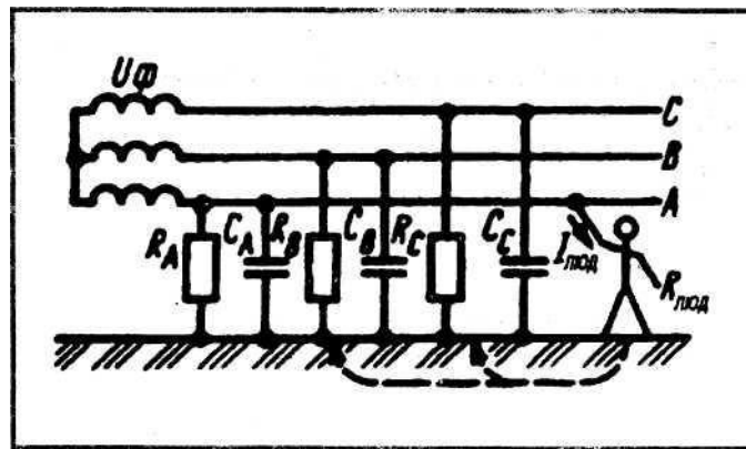
Рис. 17. Однофазне дотикання в мережі з нейтраллю, що ізолювана
