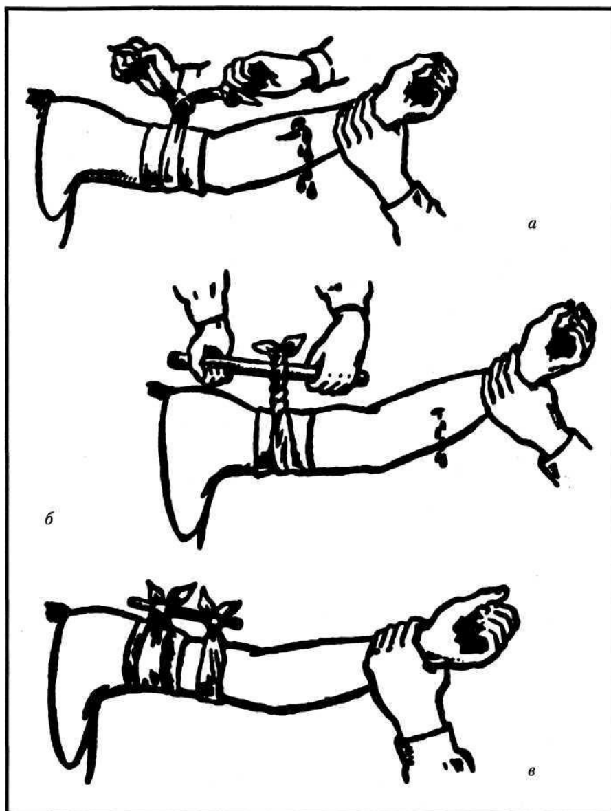
Рис. 44. Зупинка кровотечі закруткою: а) зав'язування вузла; б) закручування за допомогою палички; в) закріплення палички
