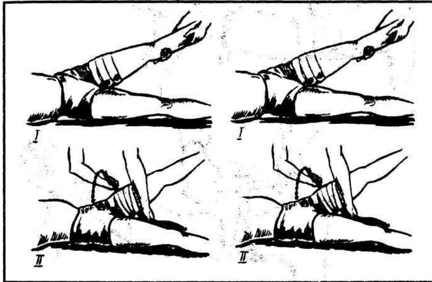
Рис. 43. Етапи накладання джгута
