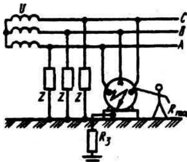
Рис. 25. Заземлення
