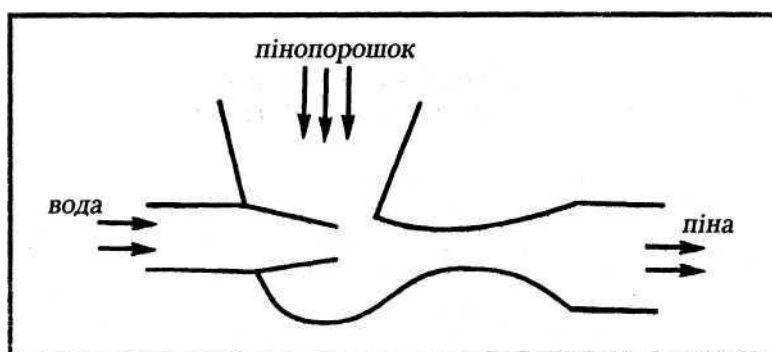
Рис. 12. Схема піногенератора
