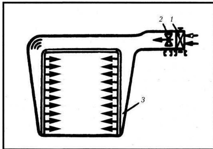
Рис. 28. Повітряно-теплова завіса з боковою подачею повітря: 1) калорифер; 2) вентилятор; 3) повітророзподільник
