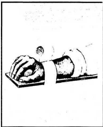
Рис. 37. Фіксація кінцівки при переломі кисті
