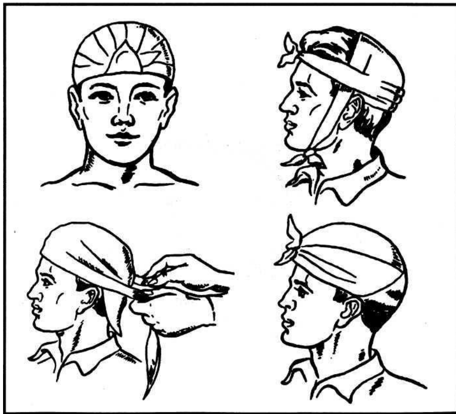
Рис. 41. Накладання пов'язки при черепно-мозковій травмі
