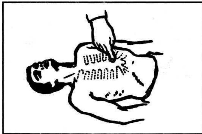
Рис. 48. Місце розташування рук при проведенні непрямого масажу серця
