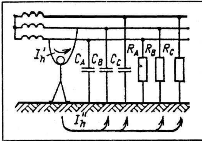
Рис. 18. Двофазне дотикання
