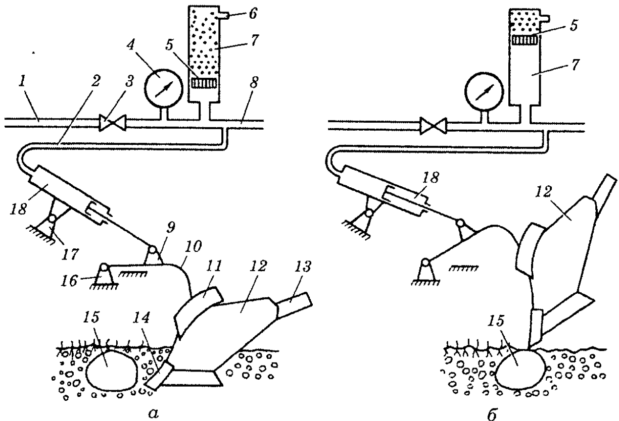
Рис.2. Схема гідропневматичного запобіжника плуга ПП-7-40:
