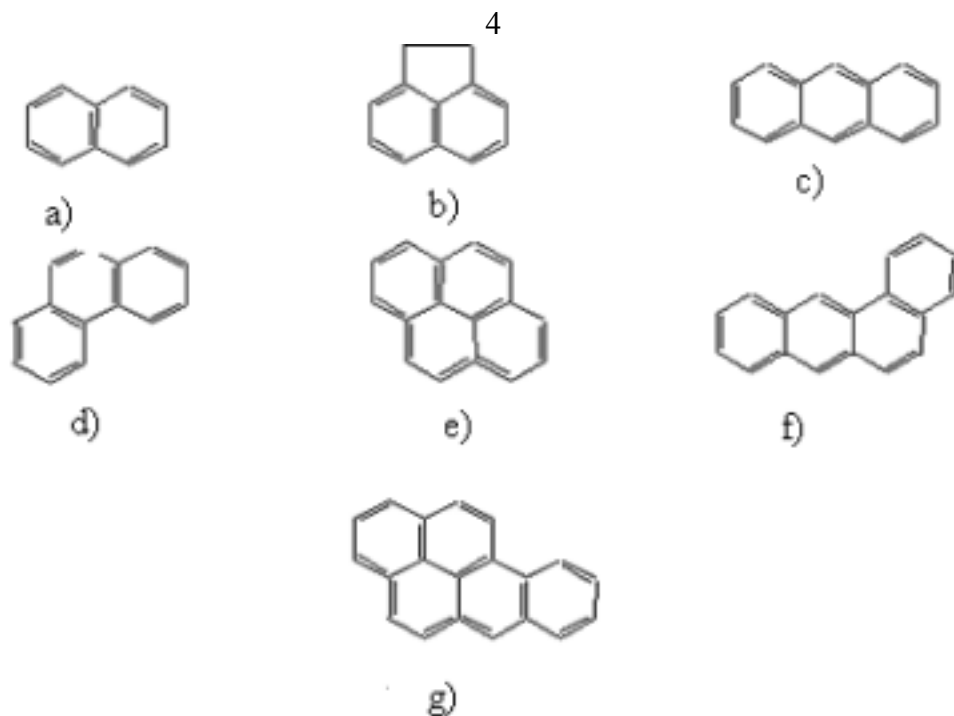
2. Irudia- Zenbait PAHren egiturak: a) naftalenoa, b) azenaflenoa, c) antrazenoa, d) fenantrenoa, e) pirenoa, f) benzo[a]antrazenoa g) benzo[a]pirenoa
