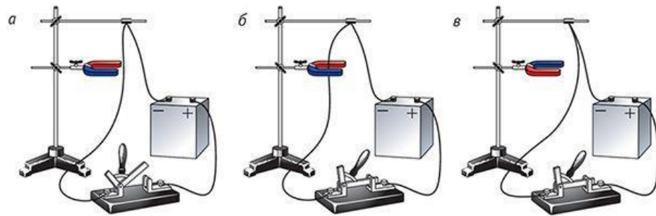
Рисунок 3 – Действие магнитного поля только на движущиеся заряды
