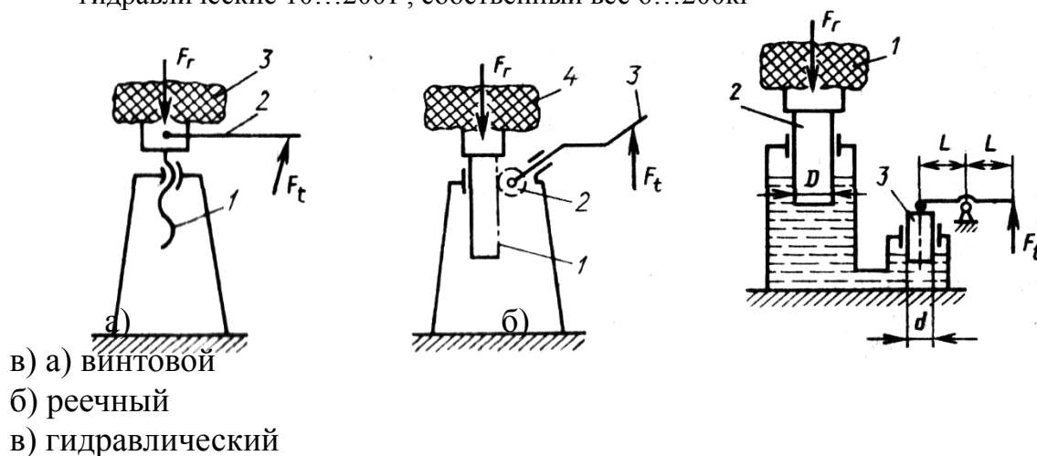
Рисунок 1 - Схемы домкратов
