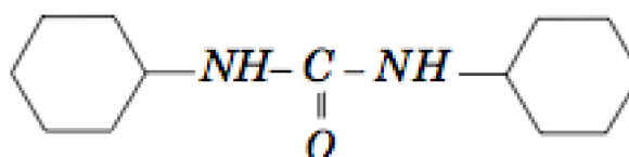
Dicyclohexylurée
