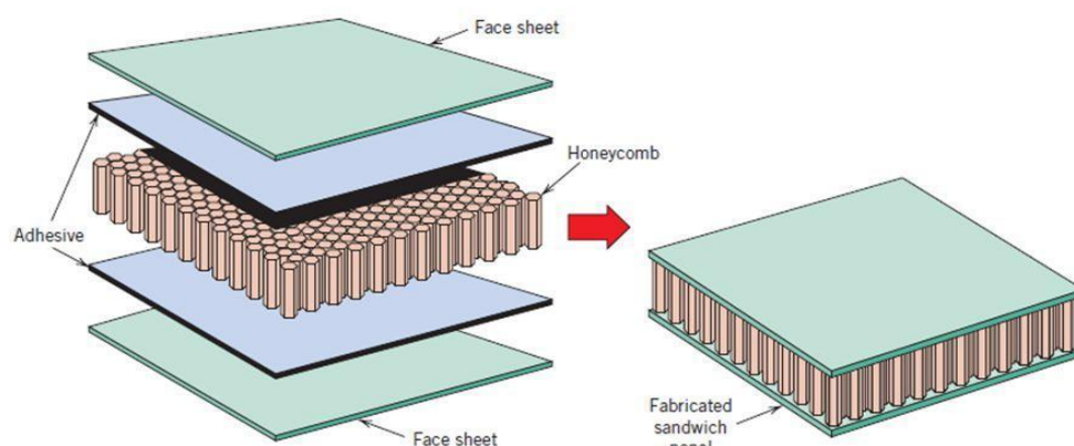
GAMBAR 1. KOMPOSIT HYBRID
