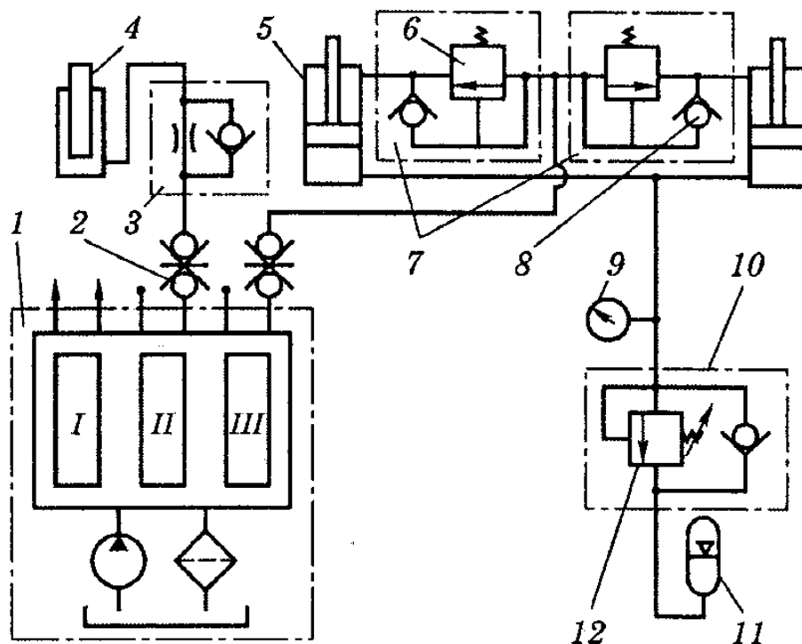
Рис. 9. Принципова схема гідроприводу рулонного преса-підбирача ПРП-1,6:
