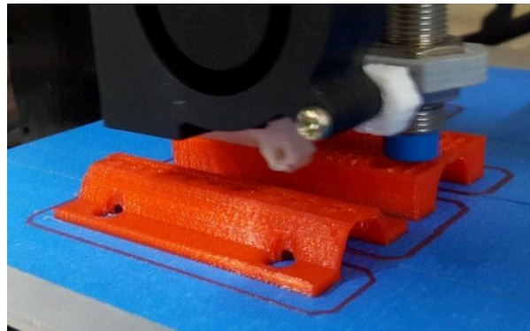
Figura 10 Vista desde la derecha de la impresión 3D de las piezas
