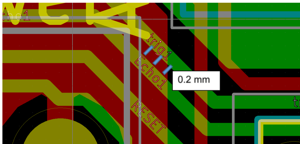
Figura 40 Dimensión entre cada pista "Clearance"
