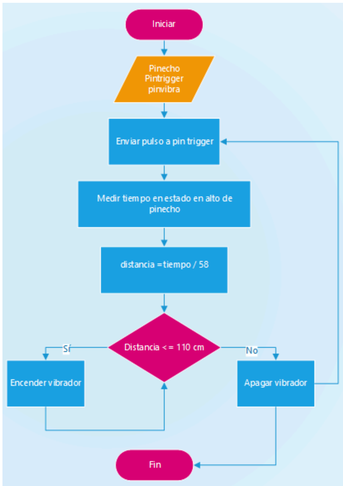
Figura 48 Algoritmo del código
