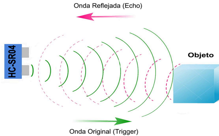
Figura 35 Forma de onda en la que detecta objetos el sensor
