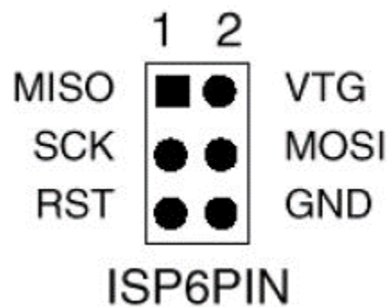
Figura 46 Configuración de pines ISP de 6
