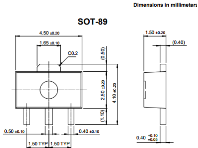
Figura 31 Empaqueta del regulador de voltaje
