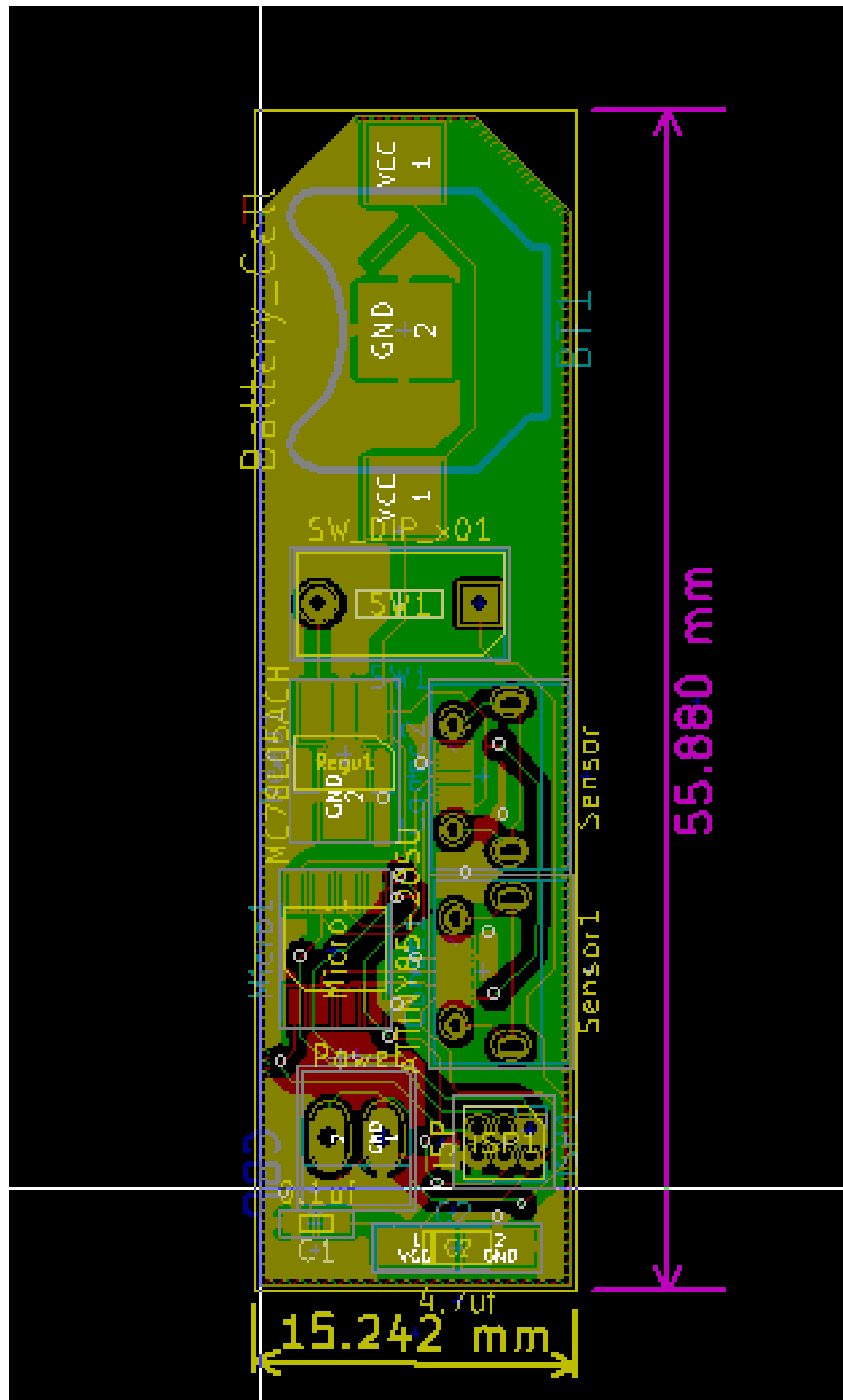
Figura 38 Diseño final de PCB echo en KICAD
