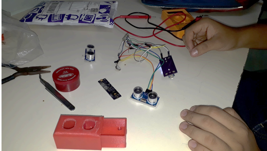
Figura 15 Prueba final de tarjeta, sensor y vibrador
