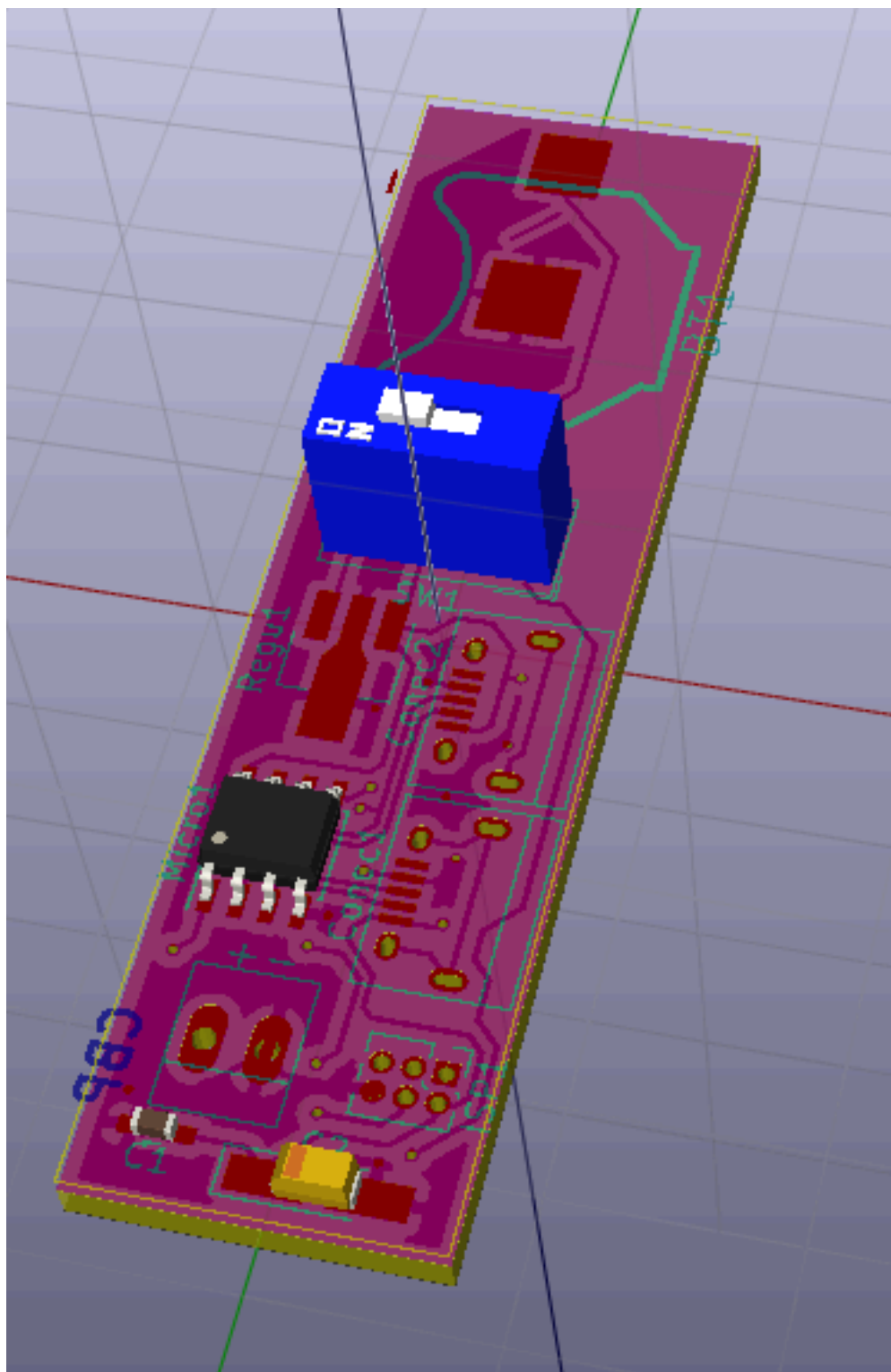
Figura 42 Diseño final de PCB vista en 3D
