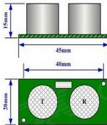
Figura 34 Diagrama del tamaño del empaquetado
