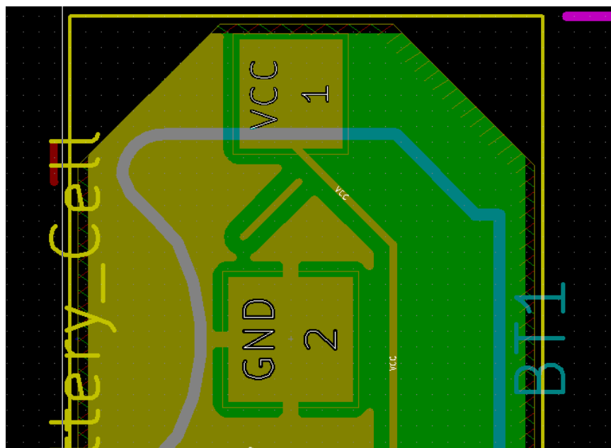
Figura 41 Figura de PCB, ubicación de batería
