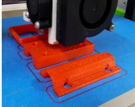
Figura 11 Vista desde la izquierda de la impresión 3D de las piezas
