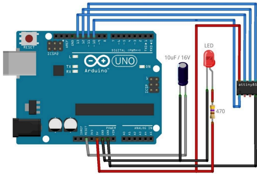
Figura 47 Conexiones ISP para programar attiny85
