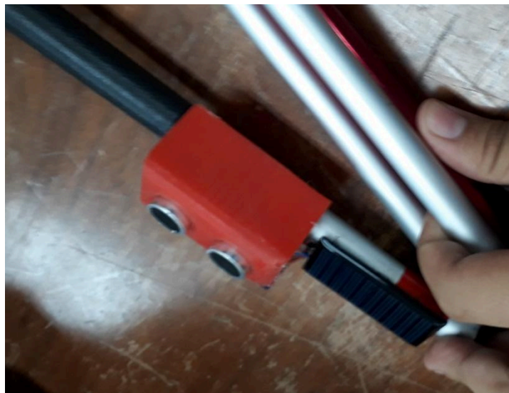
Figura 16 Integración del módulo en baston blanco
