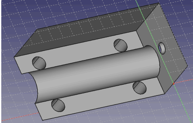
Figura 3 Vista de caja desde la parte inferior
