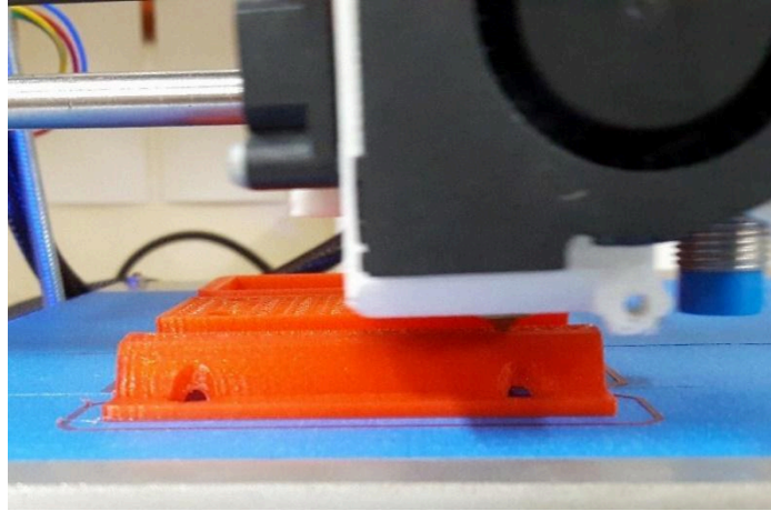
Figura 9 Proceso de impresión 3D de la placa de agarre y unión.
