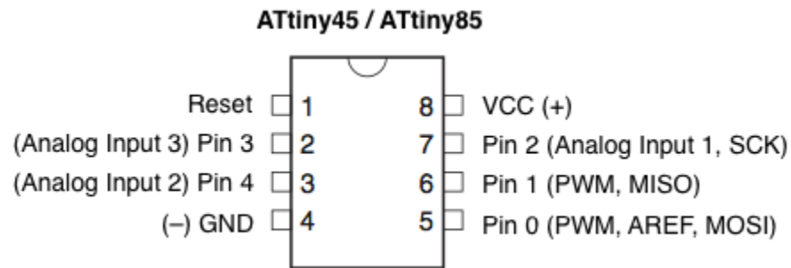
Figura 29 Configuración de pines de Attiny85
