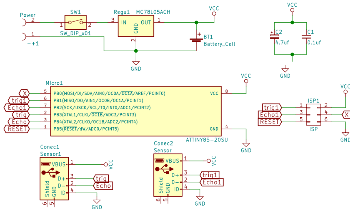
Figura 28 Esquemático de control para personas ciegas
