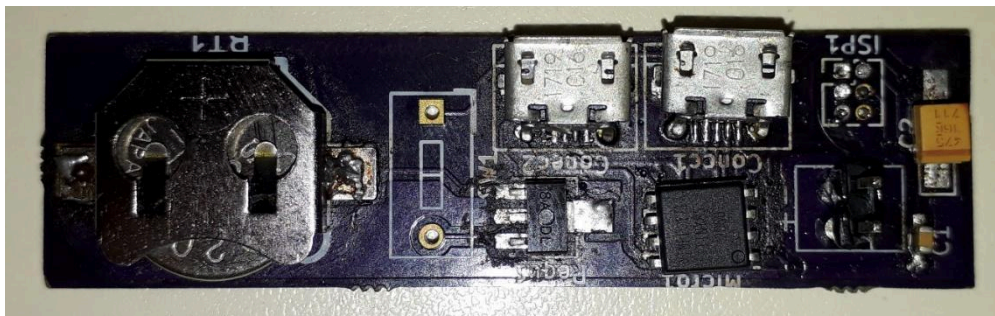
Figura 45 PCB con todos los componentes soldados
