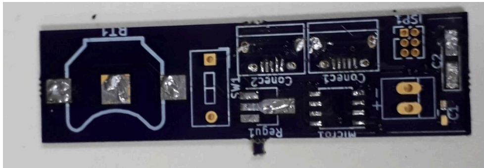
Figura 44 PCB de control con capa de estaño
