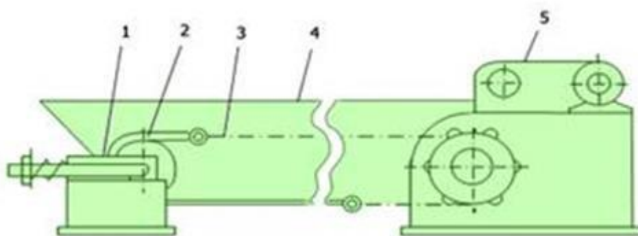
Рис. 5.10. Конструктивно-технологічна схема роздавача РВК – Ф – 74:
