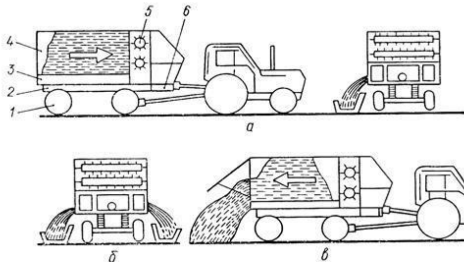
Рис. 5.4. Технологічна схема кормороздавача КТУ-10А:
