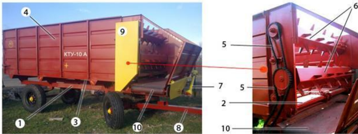
Рис. 5.3. Кормороздавач КТУ-10А:
