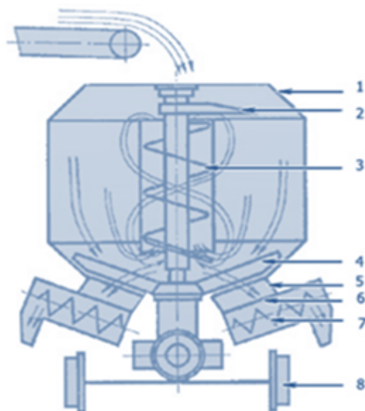
Рис. 5.13. Конструктивно-технологічна схема кормороздавача-змішувача КС-1,5:
