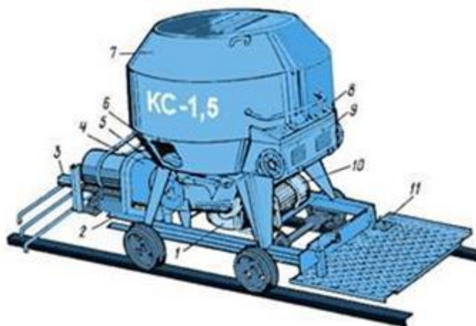
Рис. 5.12. Кормороздавач-змішувач KC-1,5:
