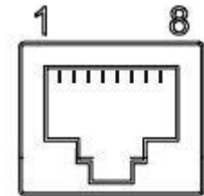
RS-422/485
