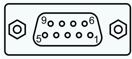
RS-232
