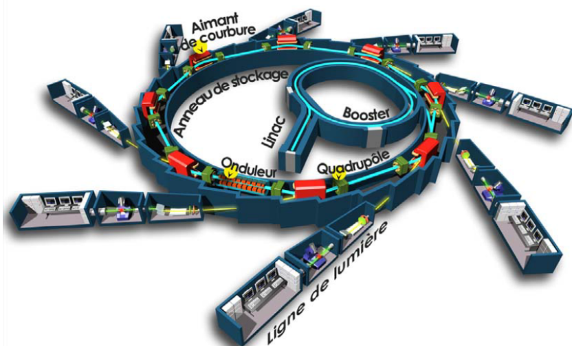
Schéma de principe d'une machine synchrotron
