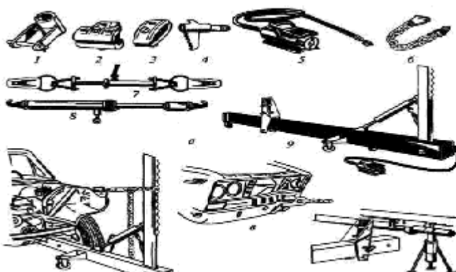
Рис. 4. Пристосування для виконання правки деформованого кузова:
