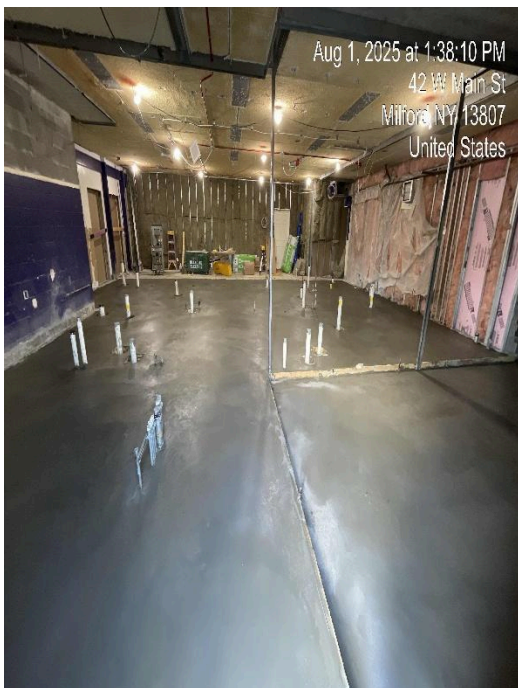
New Kitchen Slab Pour
