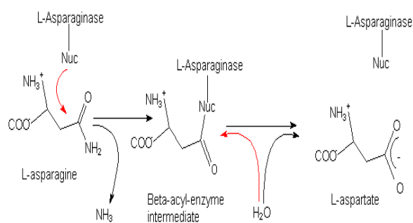
Gambar 1. Mekanisme konversi asparagin menjadi aspartat oleh asparaginase (Yadav et al. 2014). (9 pt)
