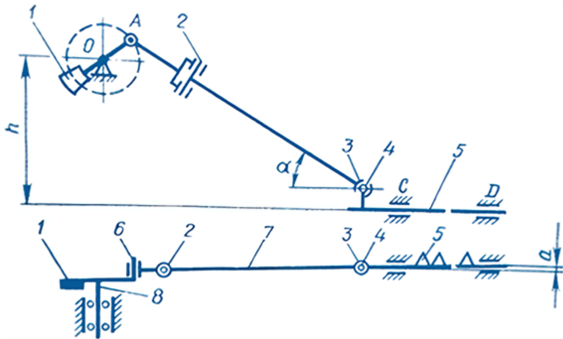
Рис. 5.2.4. Кінематична схема карбові-гонкового механізму урухомлення різального апарата:
