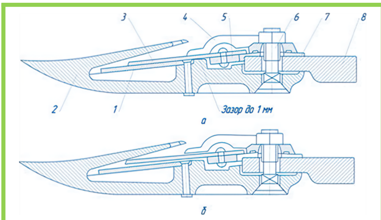
Рис. 5.2.7. Положення ножа відносно вкладиша, притискної лапки та пластини тертя:
