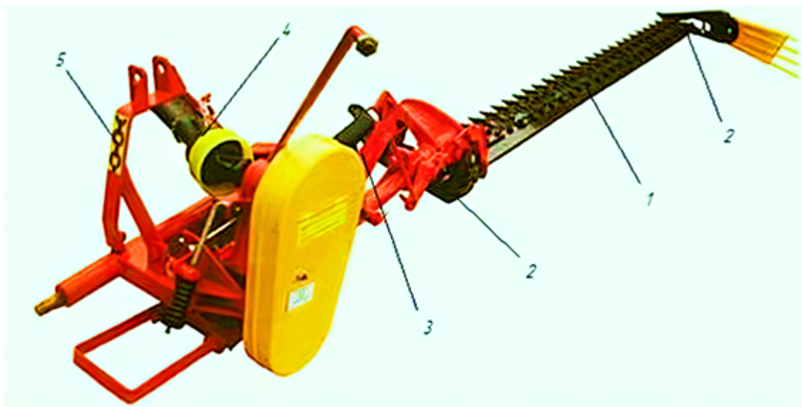
Рис. 5.2.6. Косарка сегментно-пальцева начіпна КС-Ф-2,1Б: 1 – різальний апарат; 2 – опорний башмак; 3 – механізм підйому; 4 – механізм урухомлення; 5 – начіпний механізм
