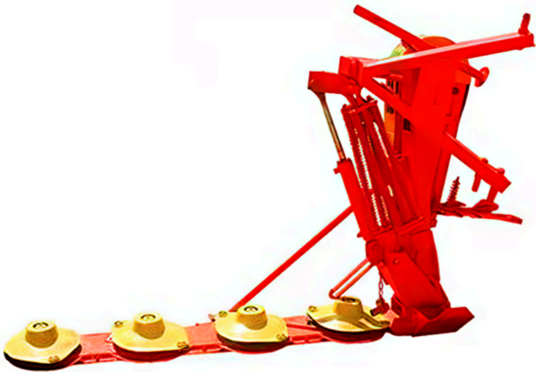
Рис. 5.2.10. Загальний вигляд косарки ротаційної однобрусної КРН-2,1А
