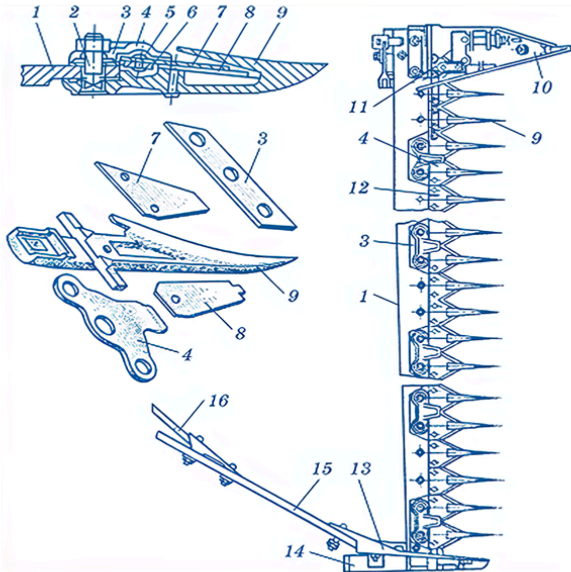
Рис. 5.2.1. Різальний апарат косарки:
