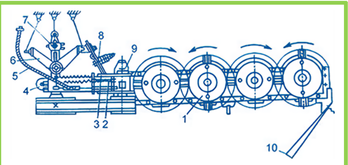
Рис. 5.2.11. Конструктивна схема косарки КРН-2,1А:
