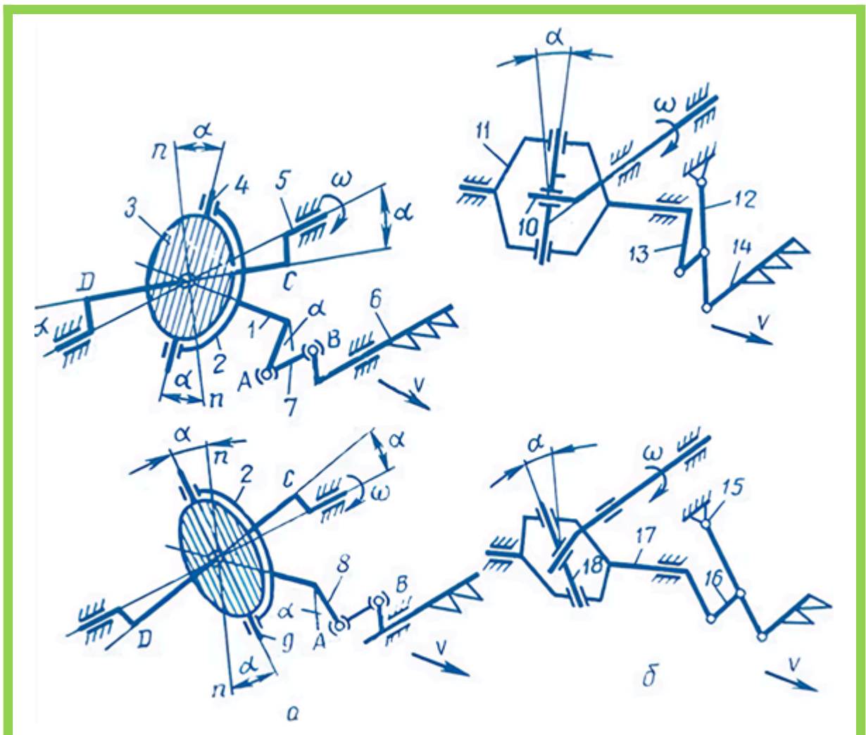
Рис. 5.2.5. Схеми механізмів урухомлення ріжучих апаратів:
