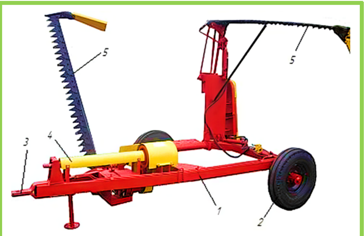
Рис. 5.2.8. Косарка двобрусна причіпна КРФ-4М: 1 – рама; 2 – ходові колеса; 3 – причіпний пристрій; 4 – карданний передавач з трансмісією; 5 – різальний апарат
