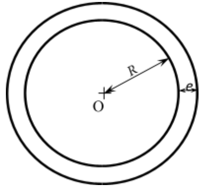
Figure 2. Transport en géométrie sphérique
