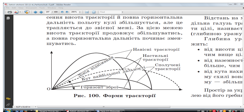
Рис. 100. Форми траєкторії
