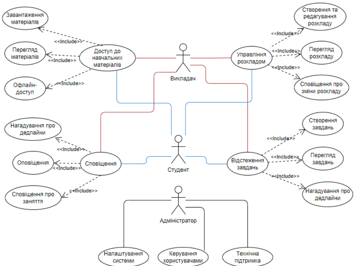
Рисунок 1.3 Діаграма варіантів використання (Use case diagram)
