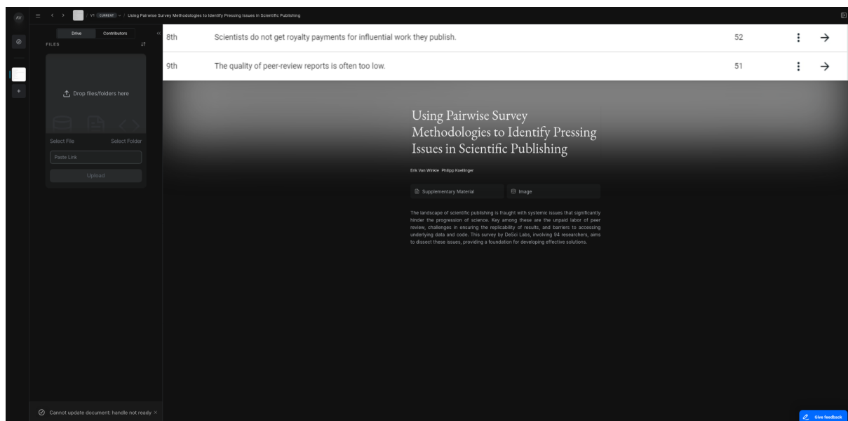
Fig. 4. Web frontend
