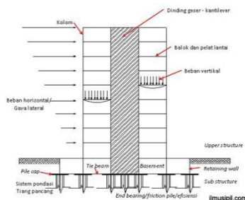
Gambar 1. Pembebanan pada Gedung bertingkat Sumber: Siho (2024)
