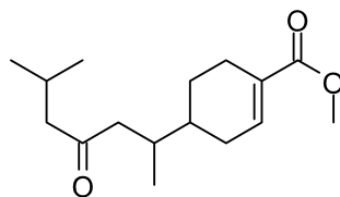
Juvabione
