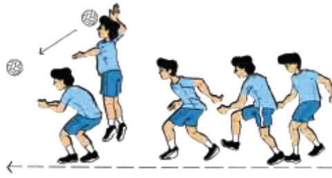
Gambar 2.6 Pembelajaran spike
